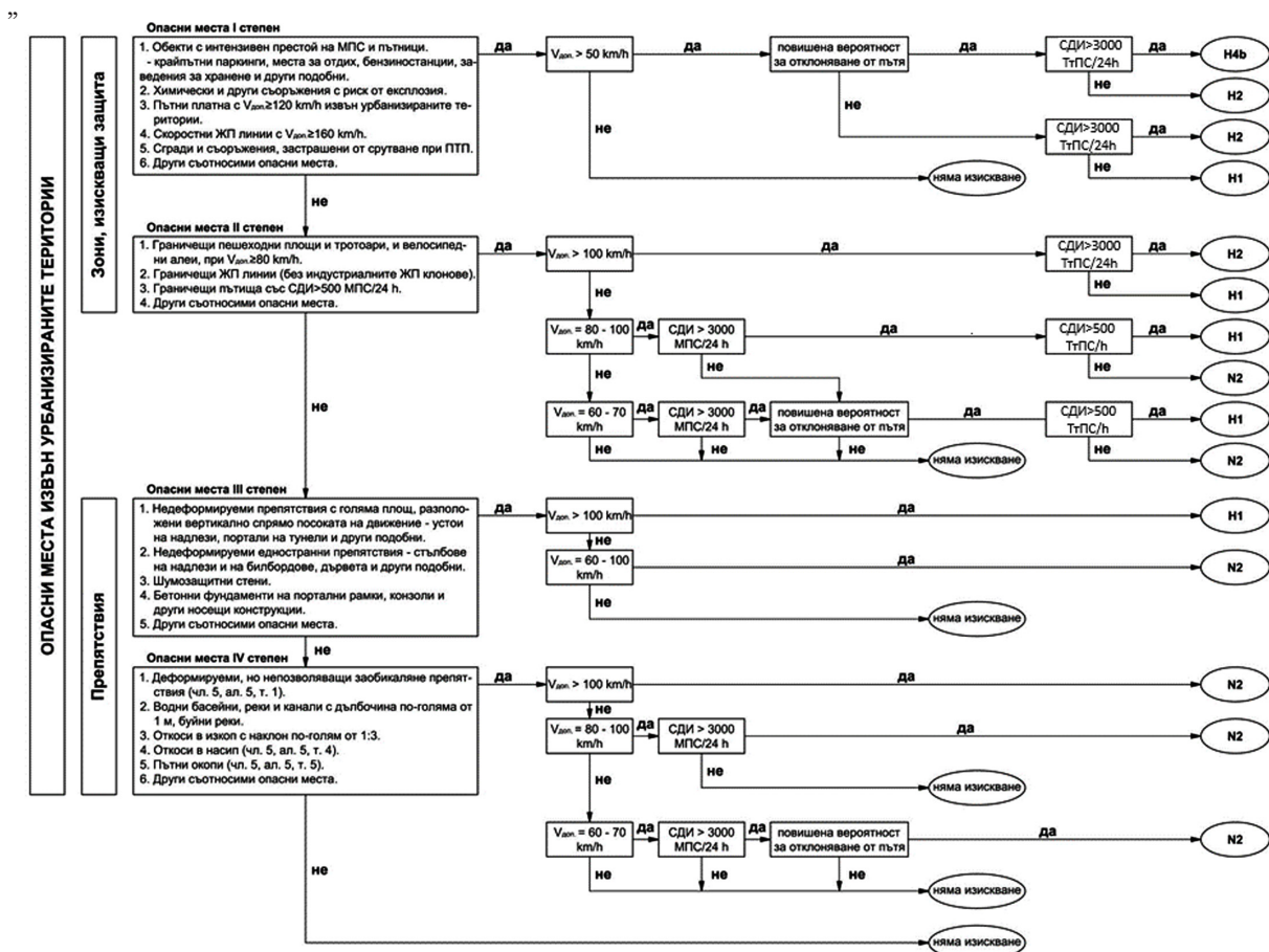
Фиг. 3. Алгоритъм за определяне на степента на задържане на ограничителна система за пътища извън населените места“.
