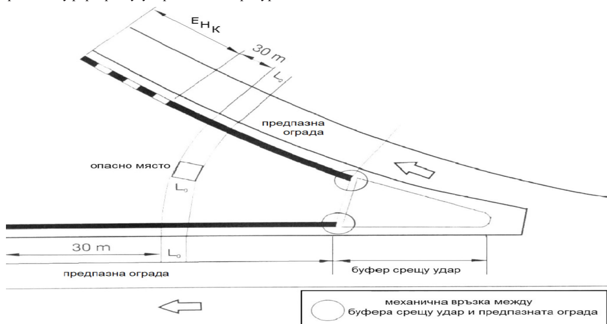
Фиг. 13. Буфер срещу удар на върха на разделителен остров пред опасно място при разделяне на големи транспортни потоци
