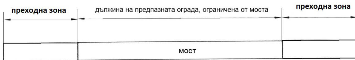
Фиг. 25. Дължини на предпазната ограда върху мост и върху мост с преходна зона
