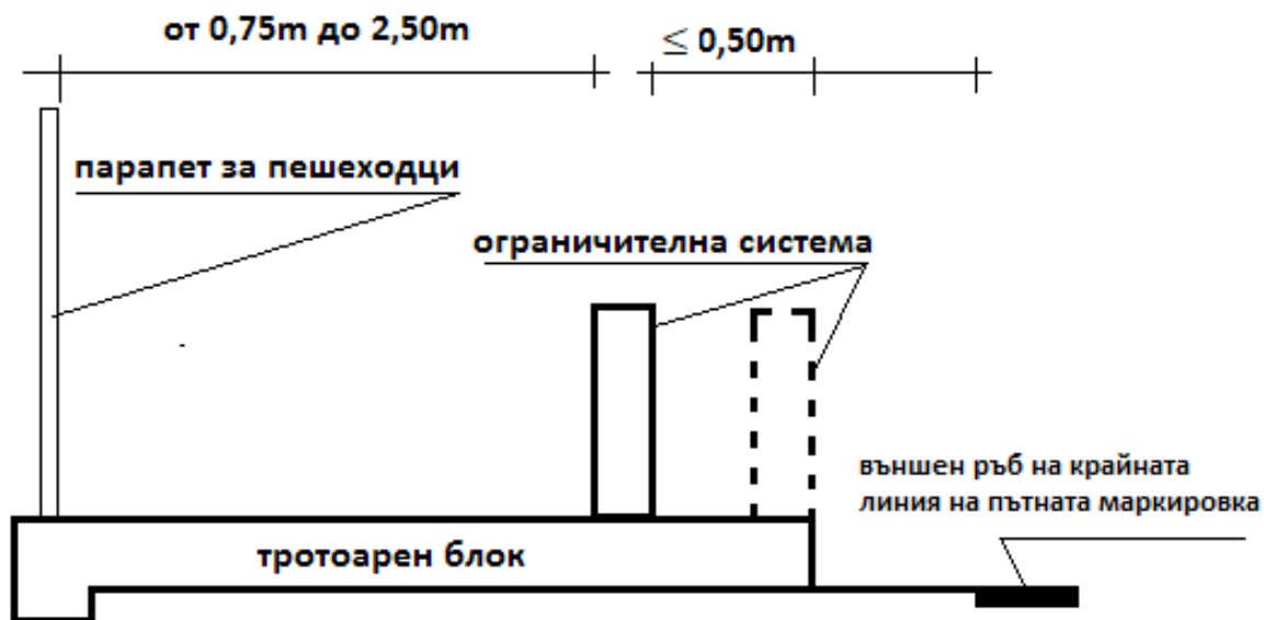
Фиг. 23. Място на ограничителна система върху тротоарен блок на съоръжение
