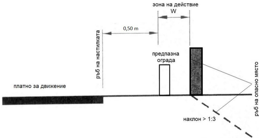
Фиг. 2. Зона на действие на ограничителна система за пътища и разстояние до платното за движение
