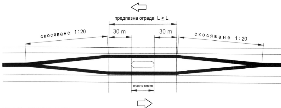
Фиг. 19. Оформяне на ограничителна система за пътища при опасно място в средна разделителна ивица
