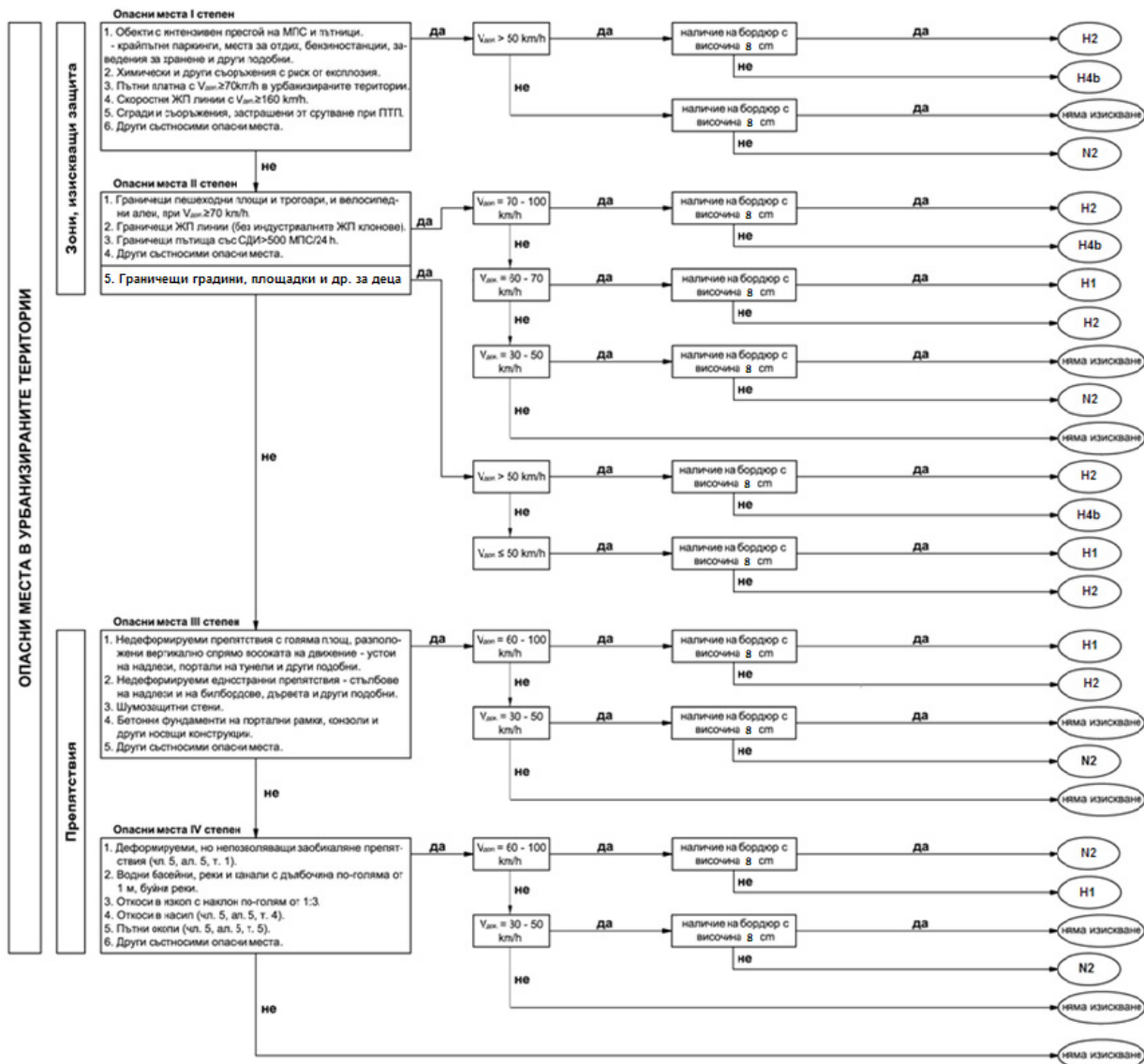
Фиг. 14. Алгоритъм за определяне на степента на задържане на ограничителна система за пътища в населени места
