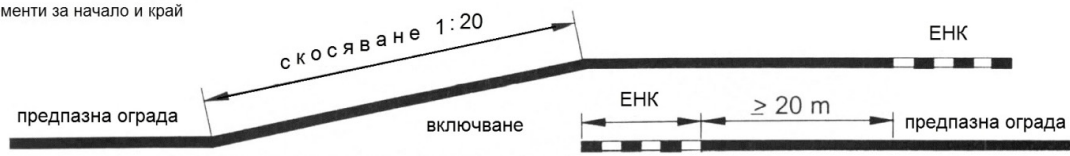
Фиг. 8. Прекъсване на ограничителна система за пътища при паралелно включване
