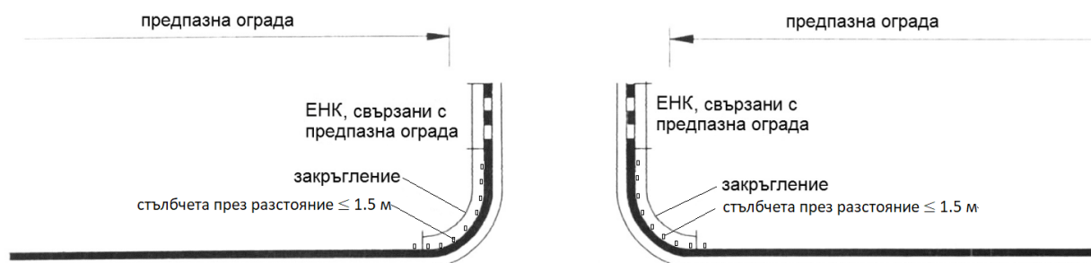
Фиг. 9г. Прекъсване на предпазната ограда със закръгления и ЕНК
