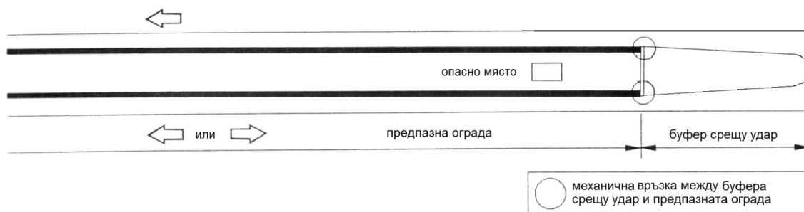
Фиг. 20. Ограничителна система, изградена двустранно в разделителната ивица от едностранна ограничителна система за пътища с буфер срещу удар за начало
