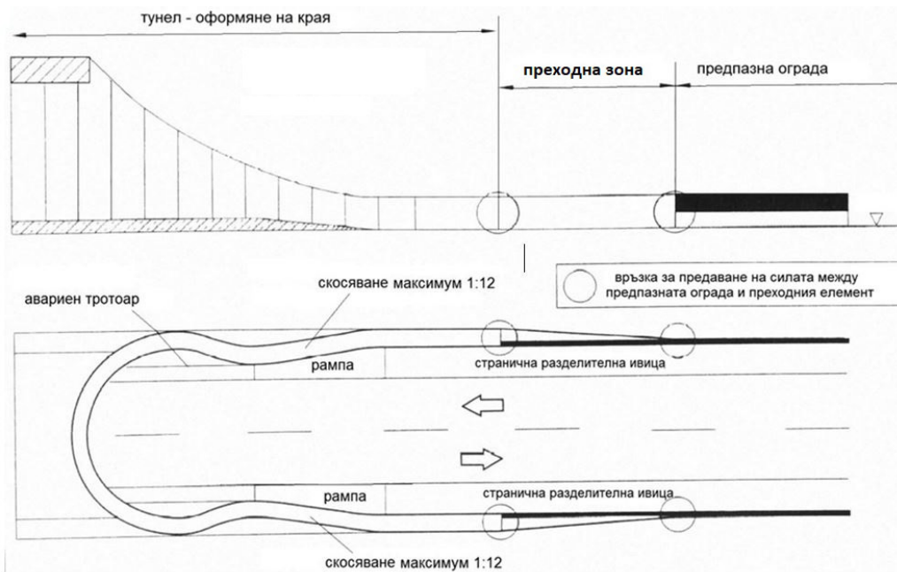
Фиг. 27. Оформяне на връзка между ограничителна система за пътища и начало на тунел
