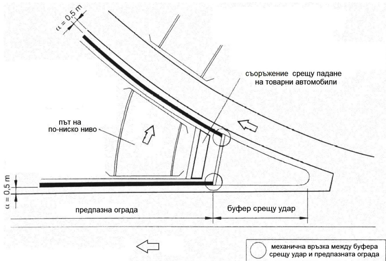
Фиг. 26. Буфер срещу удар на върха на разделителен остров върху мост
