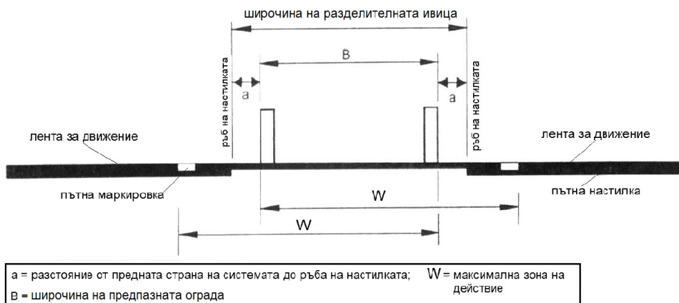
Фиг. 18. Едностранна ограничителна система за пътища с общо действие, разположена до ръба на настилката
