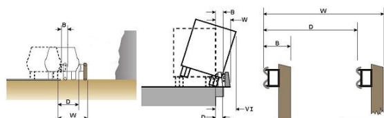
Фиг. 1. Зона на действие (W), зона на нормирано навлизане на превозното средство в незащитена зона (VI), динамична деформация на оградата (D) и широчина на оградата преди удара (B)
