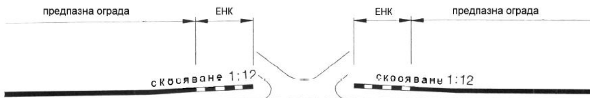
Фиг. 9а. Прекъсване на ограничителна система за пътища, скосена навън 1:12 и с елементи за зануляване
