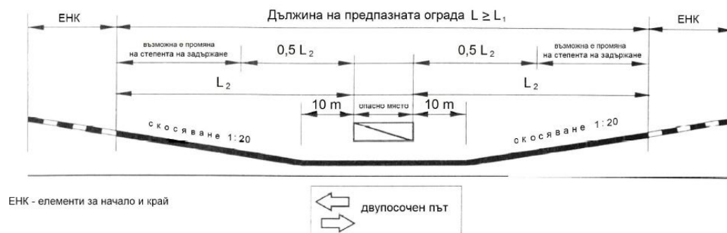
Фиг. 6. Минимална дължина на ограничителна система за пътища, изпълнена чрез двустранно скосяване преди и след опасно място при двупосочен път
