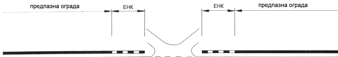
Фиг. 9б. Прекъсване на ограничителна система за пътища с елементи за начало и край
