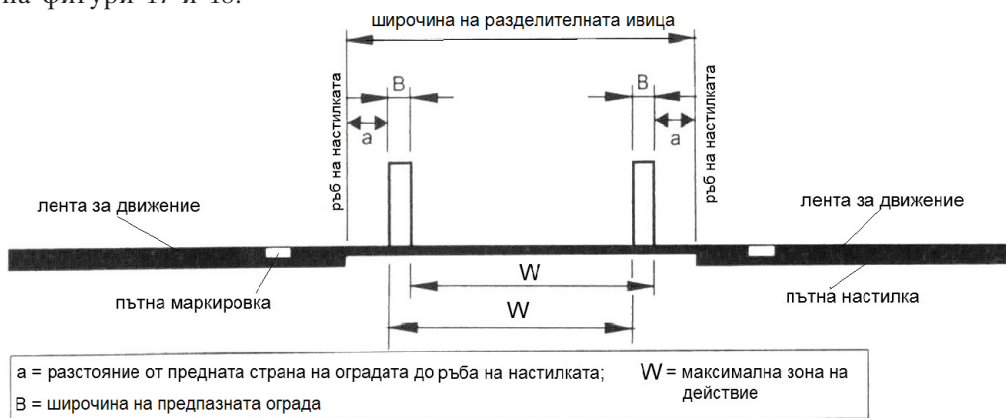
Фиг. 17. Едностранна ограничителна система за пътища с разделено действие, разположена до рѐба на настилката
