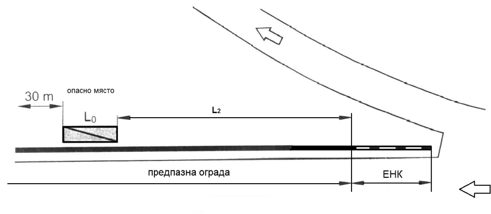
Фиг. 10. Ограничителна система за пътища с елементи за начало – зануляване при необходимо L_2 , включително при разделяне на потоци
