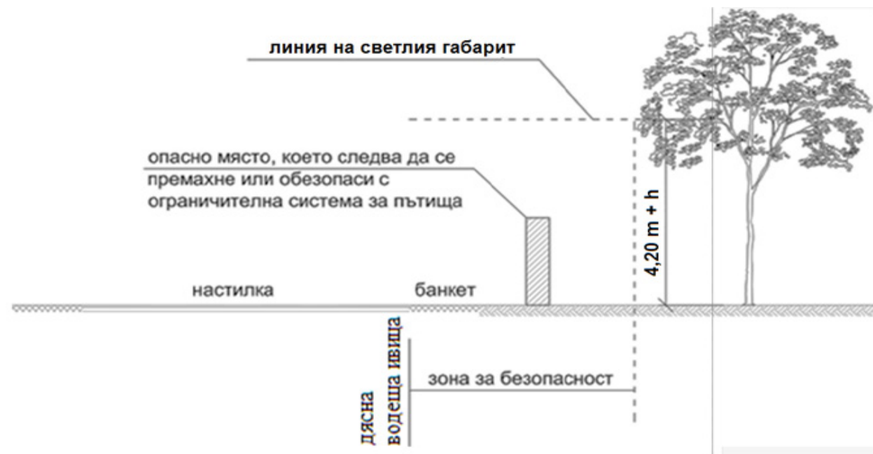
Фигура 32а. ЗБ с опасно място
