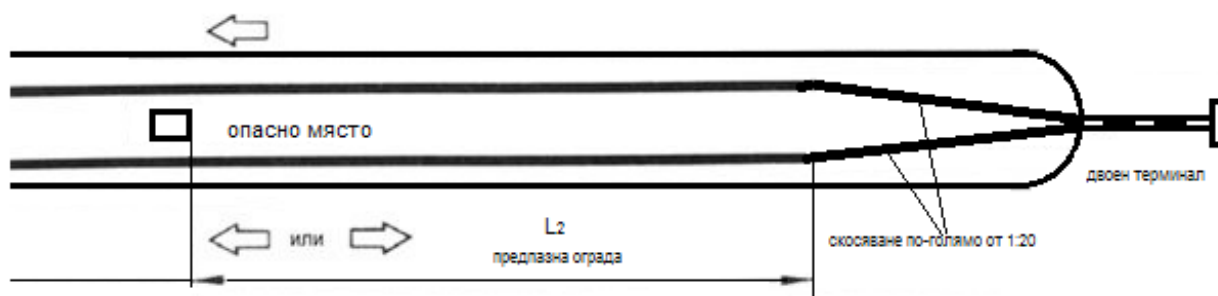
Фиг. 22. Ограничителна система, изградена двустранно в разделителна ивица от едностранна ограничителна система за пътища с начало двоен терминал
