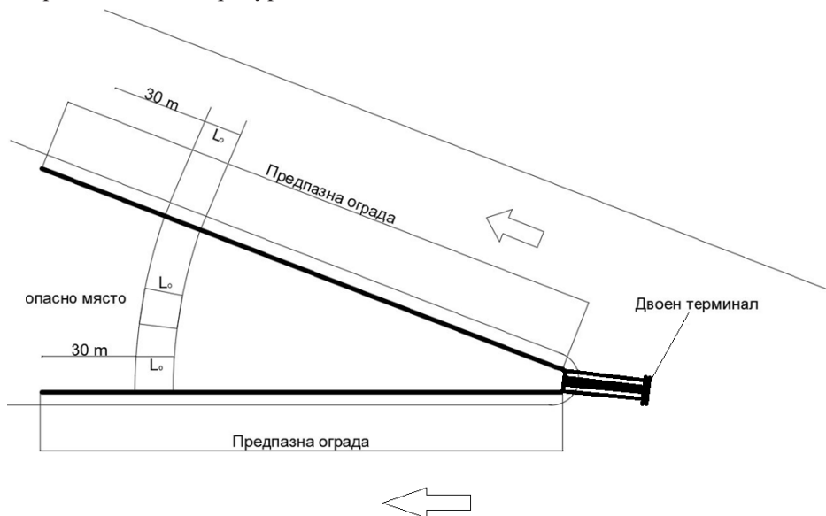
Фиг. 12. Върх на разделителен остров с предпазни огради в двете направления и елементи за начало двоен терминал
