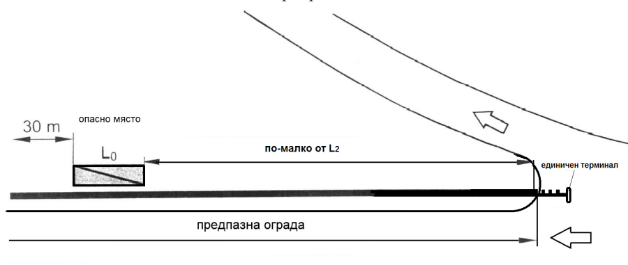
Фиг. 11. Ограничителна система за пътища с елементи за начало – единичен терминал при недостатъчно L_2 , включително при разделяне на потоци
