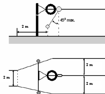
Фиг. 4. Минимална широчина и дължина на ударопоглъщаща настилка за въжени линии
