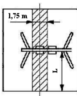
Фиг. 1. Схема на разпростиране на ударопоглъщаща настилка под седалка на люлка-махало
