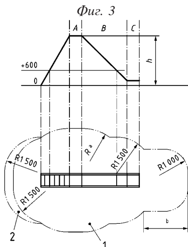
а) самостоятелна пързалка (свободно стояща пързалка)
